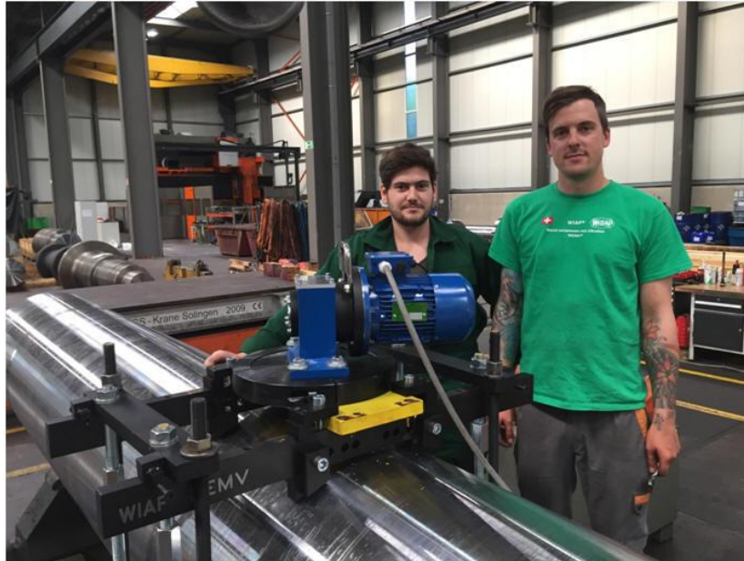
Bild 8: Aufspannvorrichtung V 20 auf Wellen bis 800 Durchmesser
